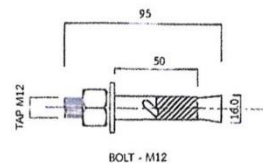
BOLT - M12
