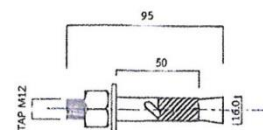
BOLT - M12
