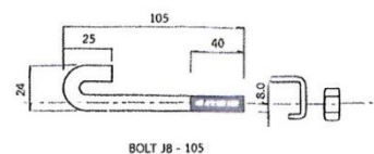
BOLT J8 - 105
