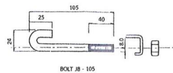
BOLT J8 - 105
